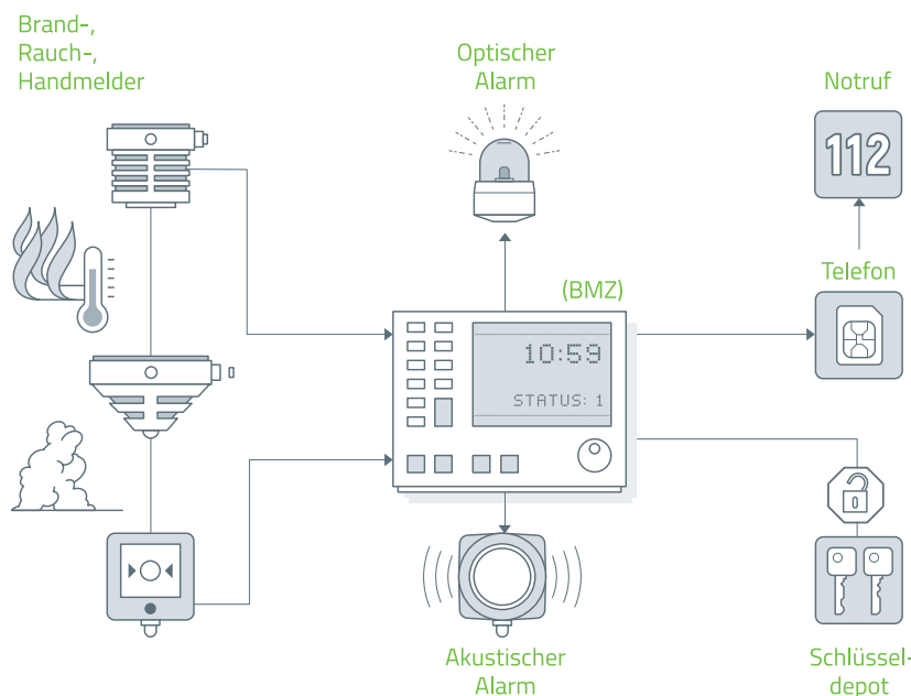
Typische Elemente einer Brandmeldeanlage mit prozessspezifischer Sensorik und angepasster Meldekette
